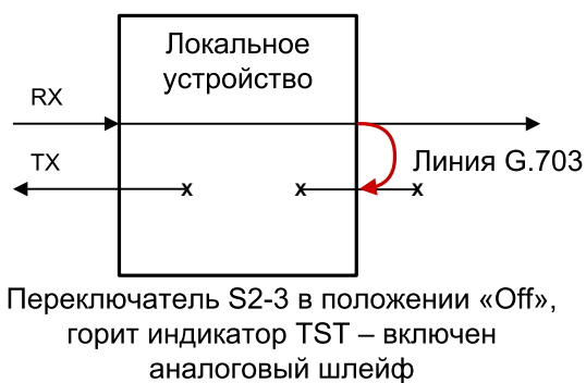
Рис. 4.3-2. Аналоговый шлейф
