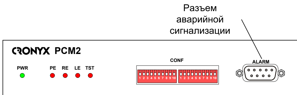
Рис. 3.3-1. Передняя панель модема PCM2/М
