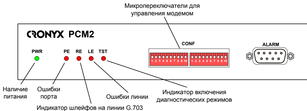
Рис. 4.1-1. Расположение индикаторов и органов управления на передней панели модема PCM2/M
