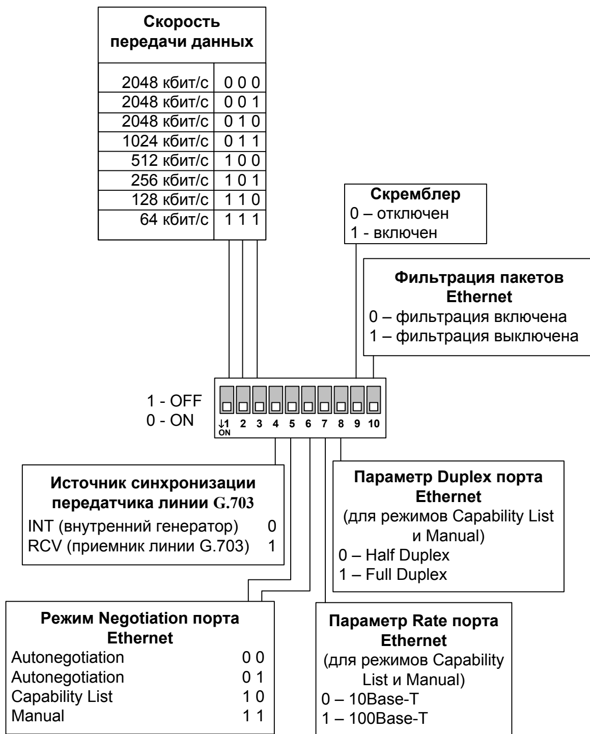
Рис. 4.1-4. Функции группы микропереключателей S1
