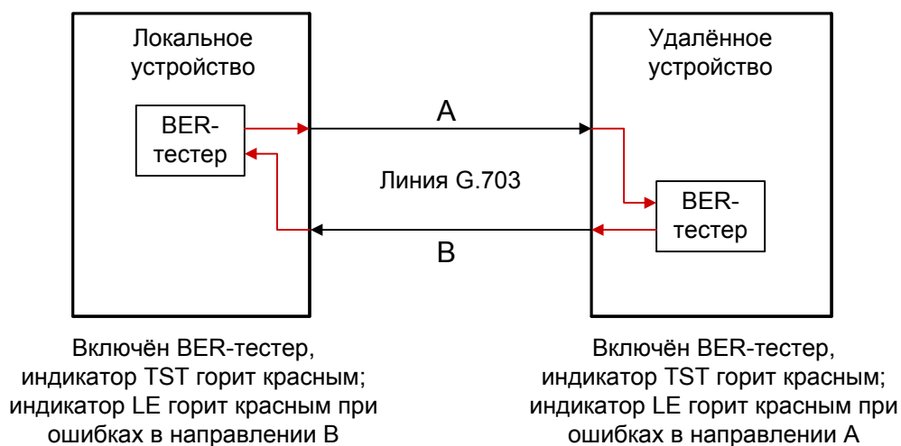
Рис. 4.4-2. Встречное включение BER-тестеров
