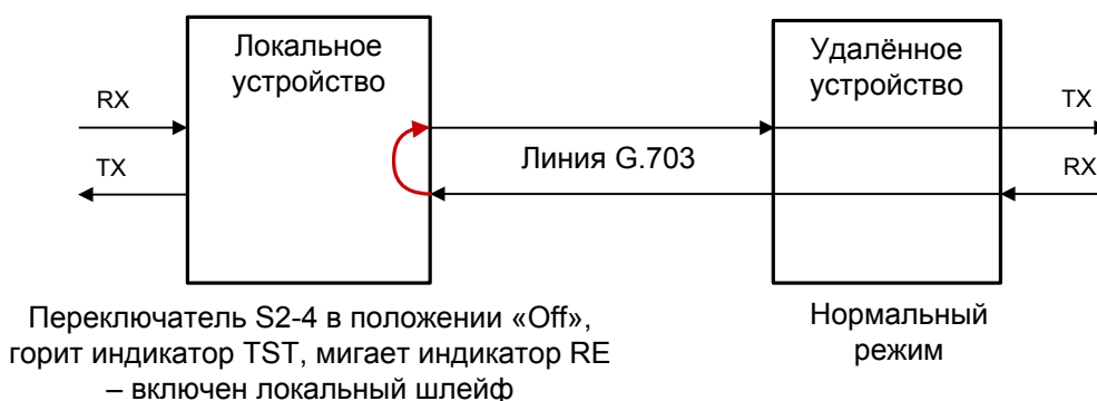
Рис. 4.3-3. Локальный шлейф на линии G.703
