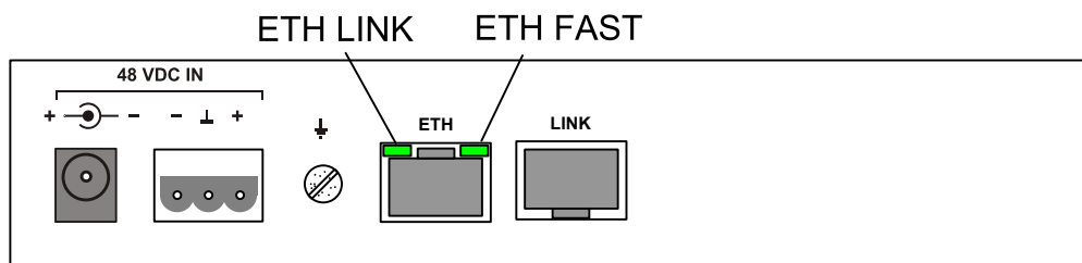
Рис. 4.1-2. Индикаторы на задней панели модема PCM2/M-ETV
