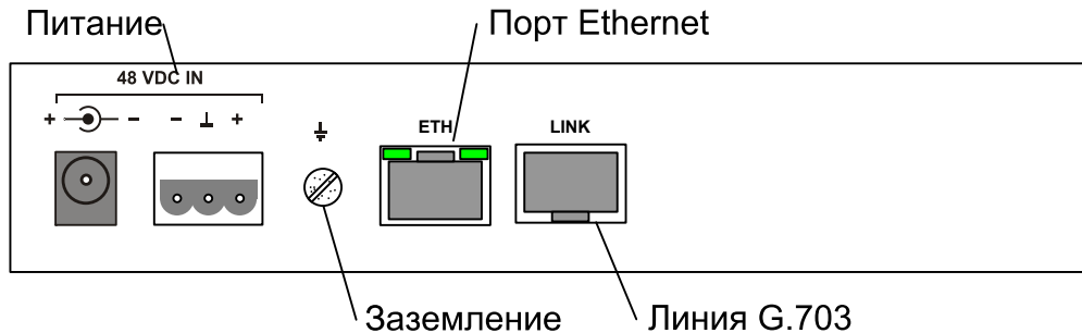
Рис. 3.3-2. Расположение разъёмов на задней панели модема РСМ2/М-ЕТV
