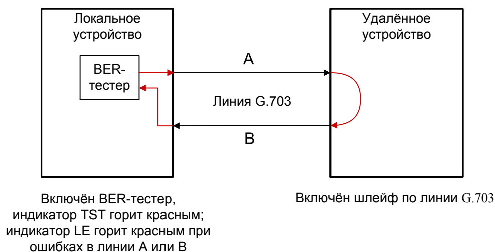
Рис. 4.4-1. Тестирование линии через удалённый шлейф
