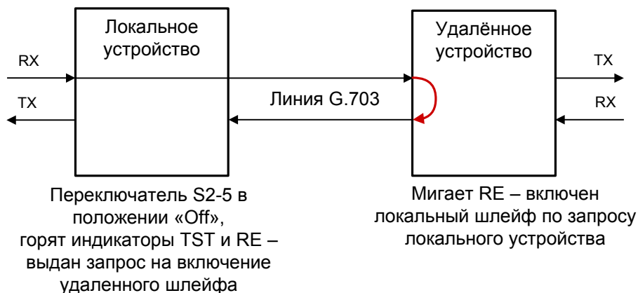
Рис. 4.3-4. Удаленный шлейф на линии G.703
