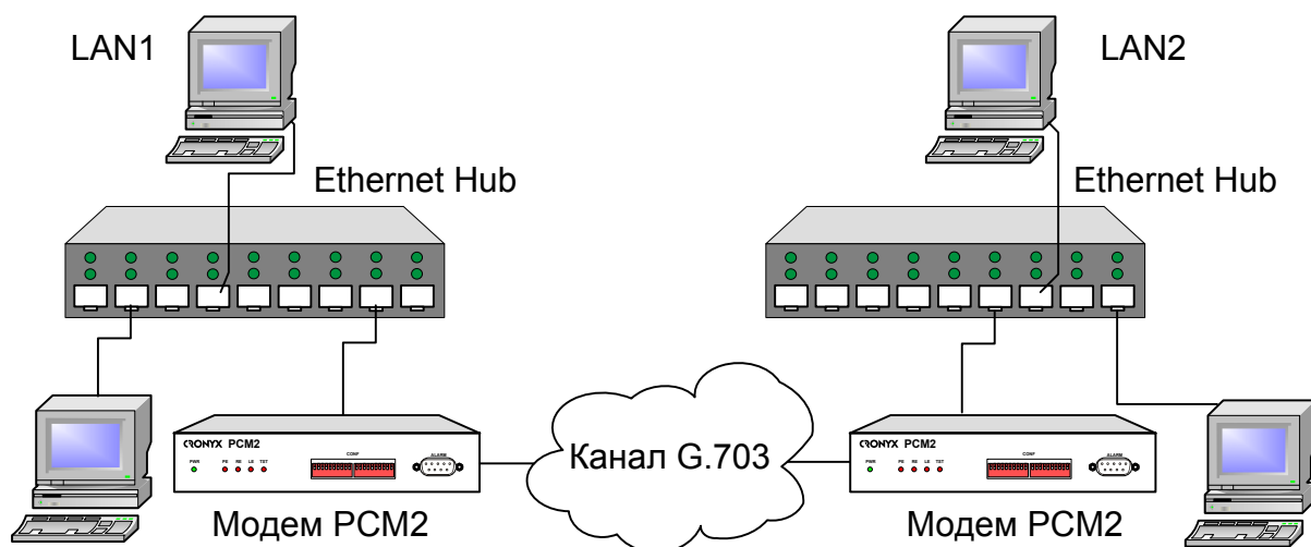
Рис. 1.1-1. Объединение локальных сетей по каналу G.703 2 Мбит/с
